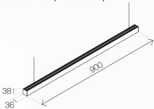
Linea sospensione con cavetti / Linea - suspension lamp
