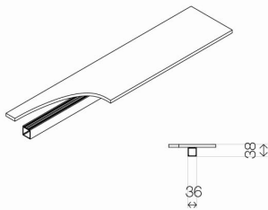
Linea fissaggio a soffitto / Linea - ceiling lamp
