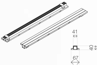
Linea fissaggio incasso / Linea - lighting recessed
